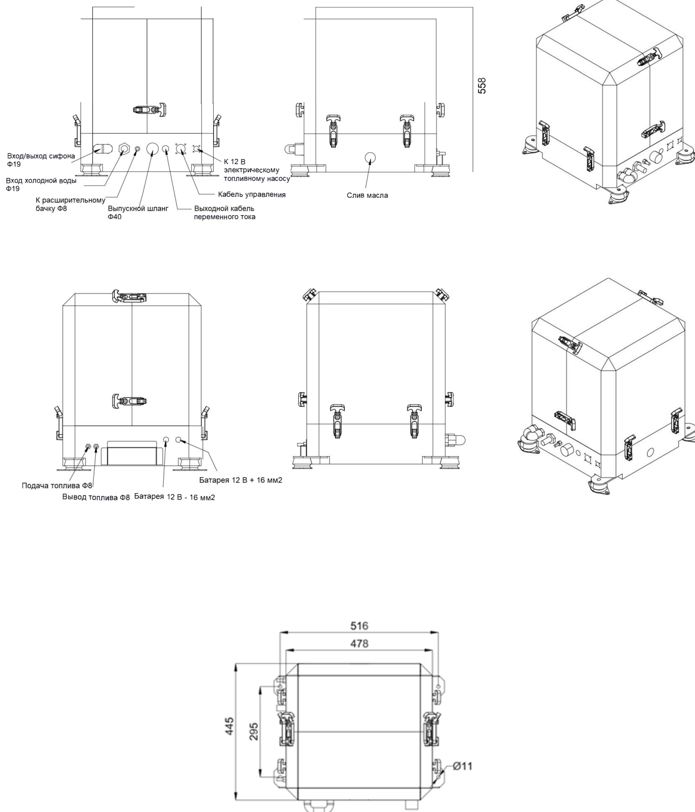
Рисунок 14: Чертежи генератора H-MG6MR/ H-MG8MR
